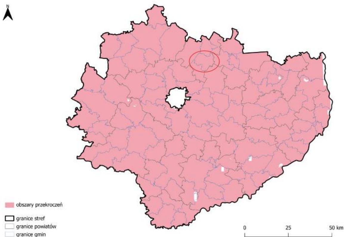
Mapa 3 Zasięg obszaru przekroczeń poziomu celu długoterminowego ozonu ze względu na ochronę roślin w województwie świętokrzyskim w 2024 roku
