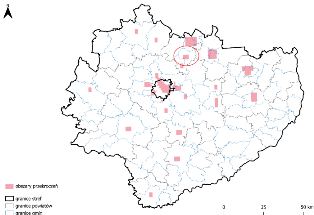
Mapa 1 Zasięg obszarów przekroczeń poziomu docelowego benzo(a)pirenu w pyłe zawieszonym PM10 określonego ze względu na ochronę zdrowia w województwie świętokrzyskim w 2024 roku
