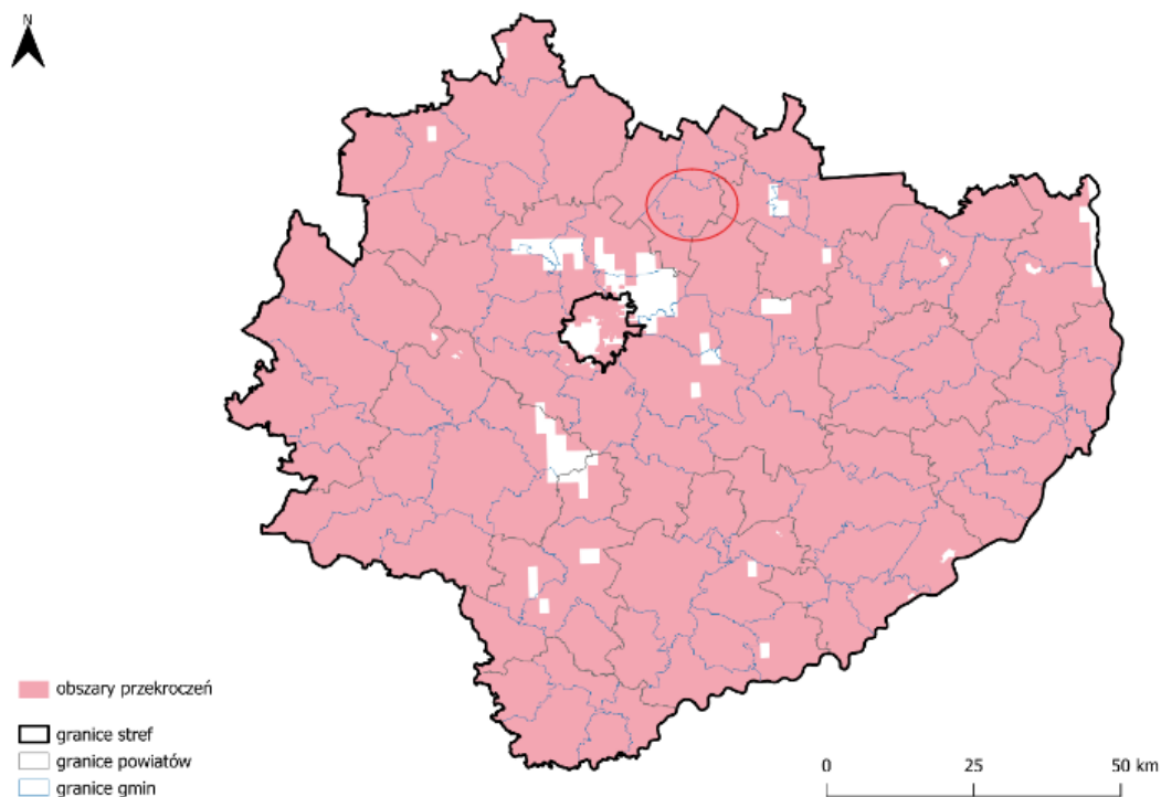
Mapa 2 Zasięg obszaru przekroczeń poziomu celu długoterminowego ozonu ze względu na ochronę zdrowia w województwie świętokrzyskim w 2024 roku
